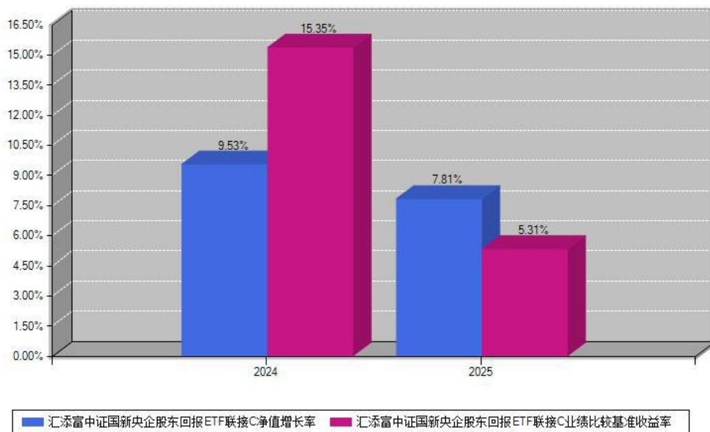
汇添富中证国新央企股东回报ETF联接C每年净值增长率与同期业绩基准收益率对比图
