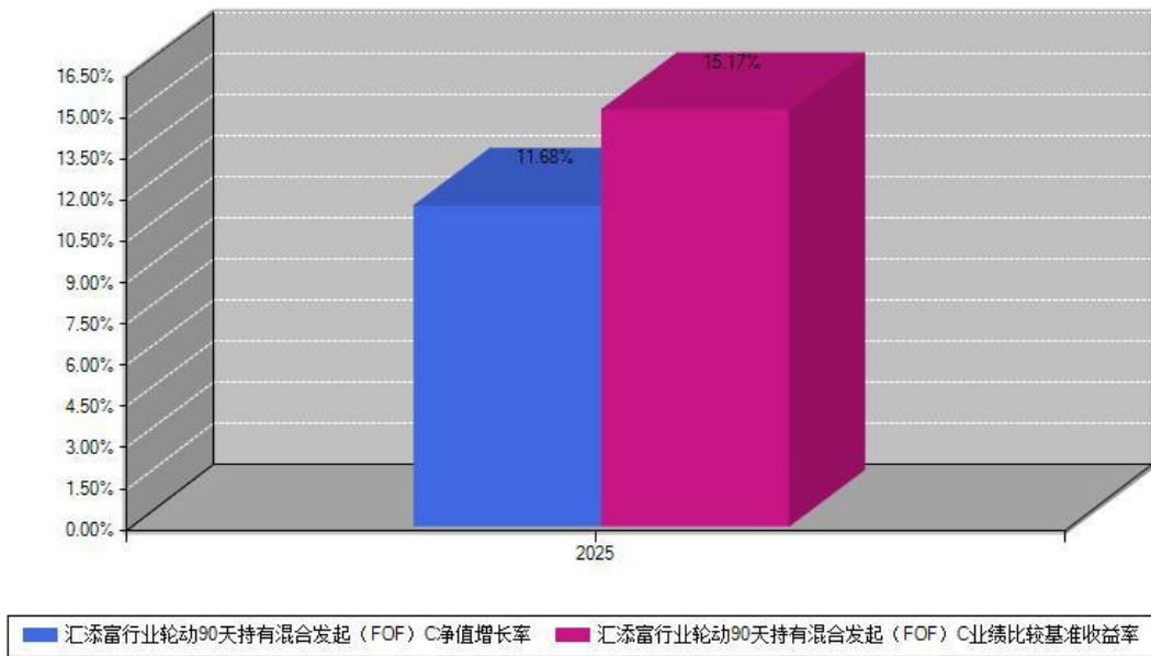
汇添富行业轮动90天持有混合发起（FOF）C每年净值增长率与同期业绩基准收益率对比图
